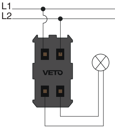
Diagrama de instalación Interruptor bipolar
