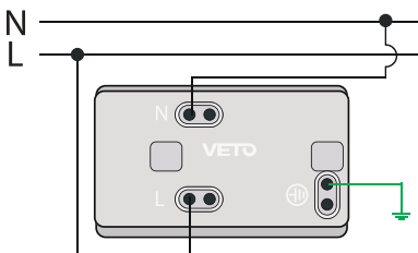
Toma doble universal 2P+E
