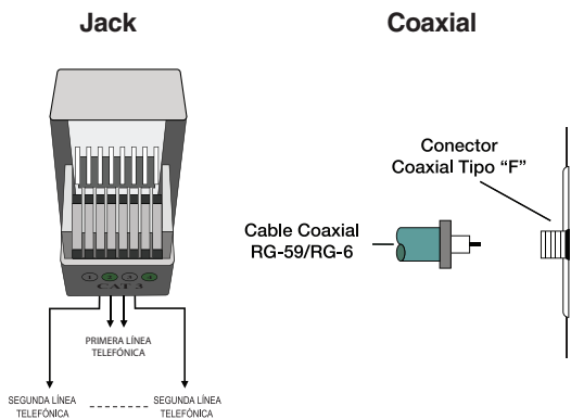
Diagrama de instalación
