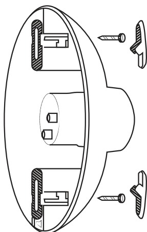
Diagrama de Instalación
