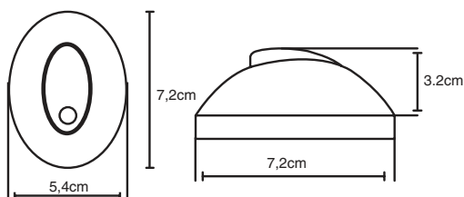
Diagrama de Instalación Pulsador
