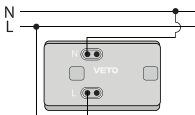
Toma universal 2P
