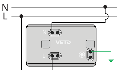
Toma doble universal 2P+E
