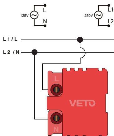
Diagrama de Instalación Base de carga USB
