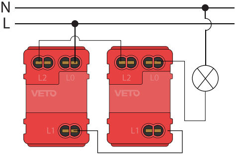
Diagrama de instalación Conmutador
