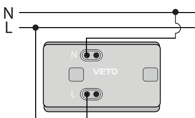
Toma doble 2P
